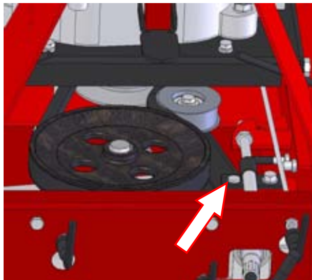
Obr. 17: Mazací místo - čep kladky spojky pojezdu
